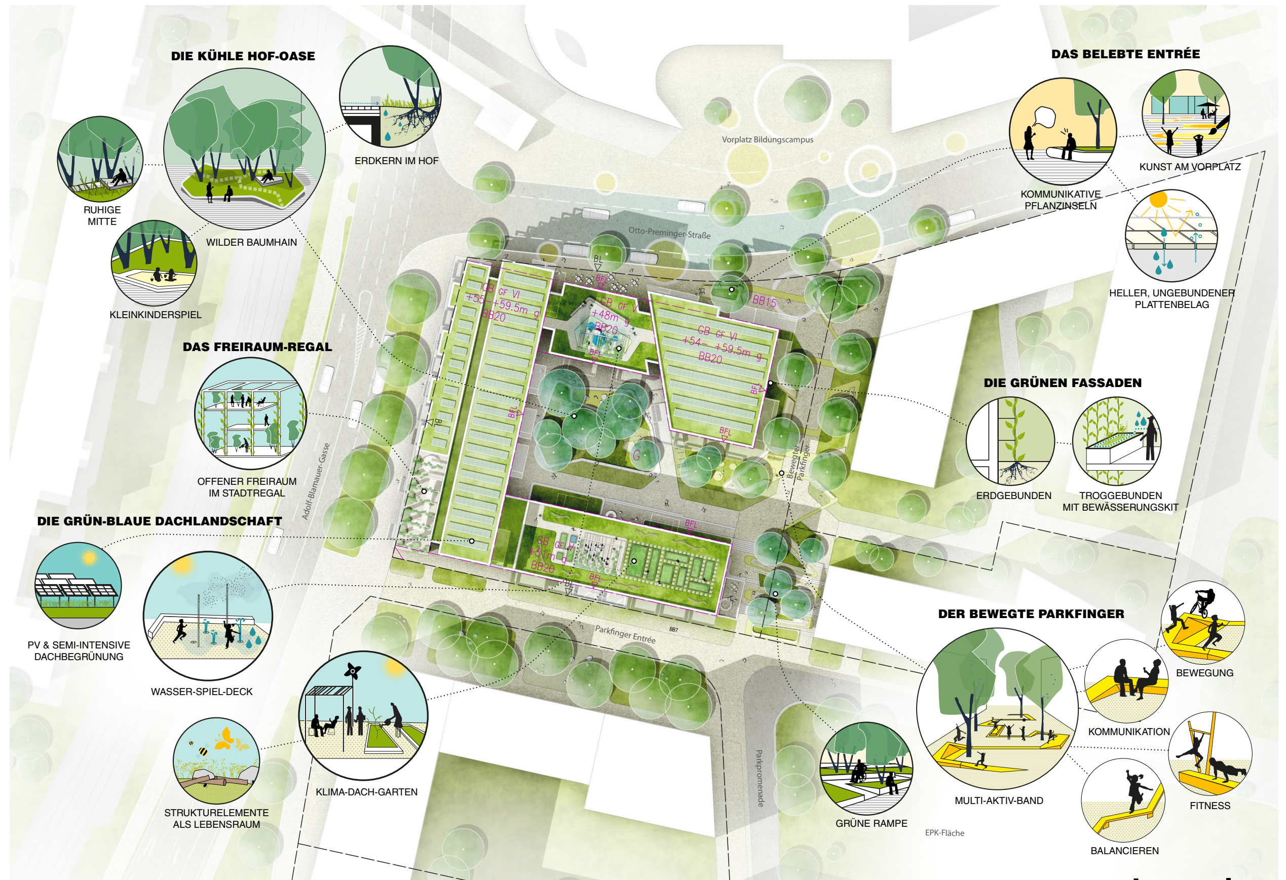
Lageplan
